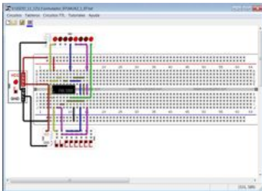
Figura 1. Circuito diseñado con el simulador "Constructor Virtual de Circuitos" [9].
